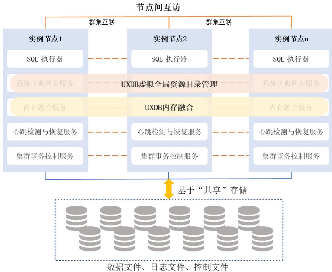
UXDB SRAC 部署示意图
